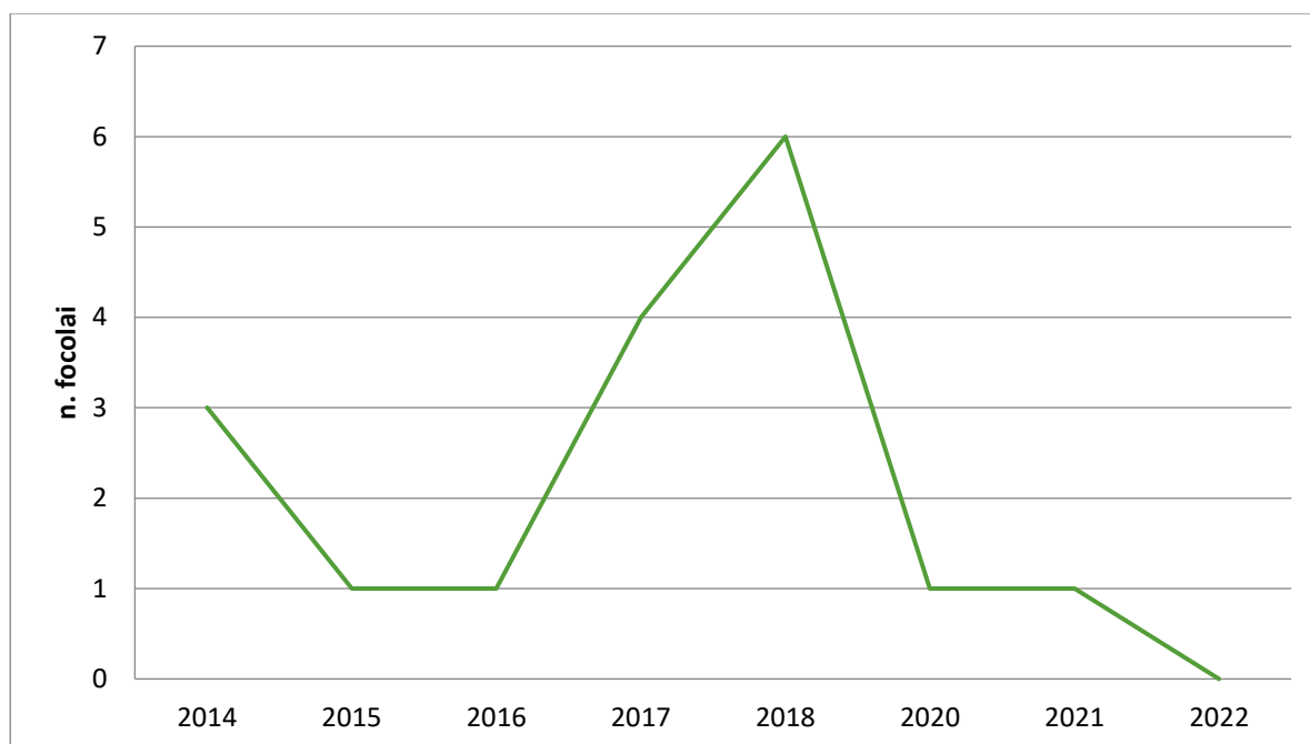
Figura 6-35: Andamento dei focolai di AIE confermati dal 2014 al 2022.
